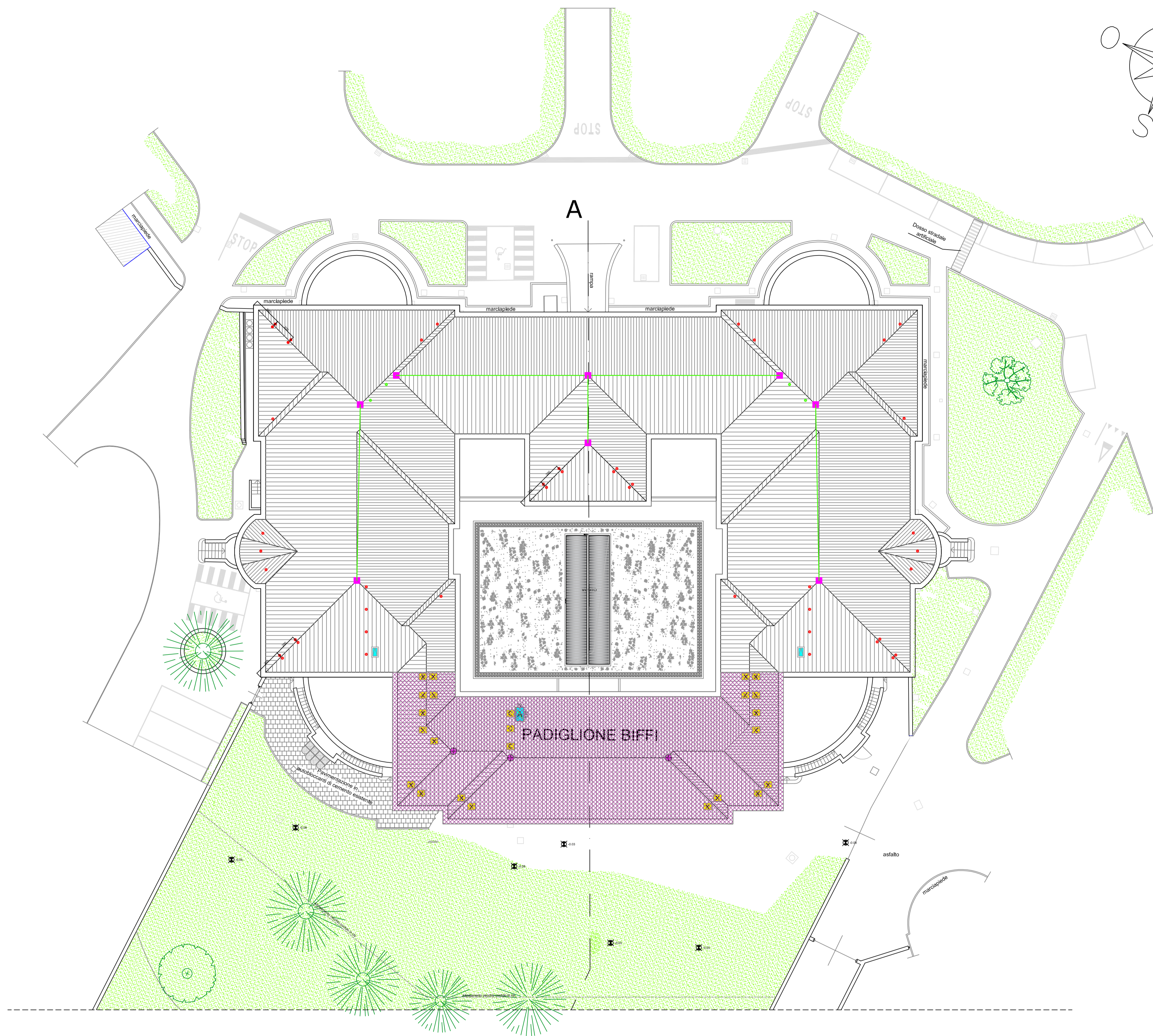
Planimetria generale Schema Linea Vita Scala 1:200
